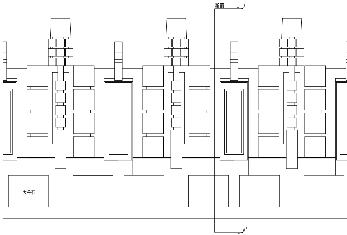
立面图
