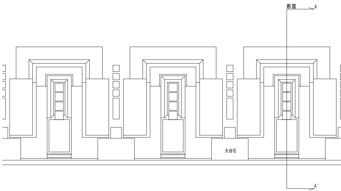
立面图
